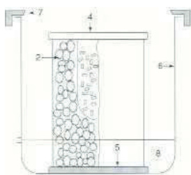
Sezione longitudinale fumigatore
